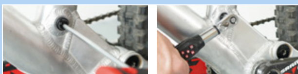
Rysunek 177: Mocowanie osi sworznia
