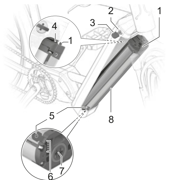
Rysunek 36: Szczegóły PowerTube 750
