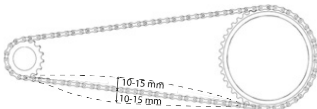
Rysunek 138: Kontrola naprężenia łańcucha
