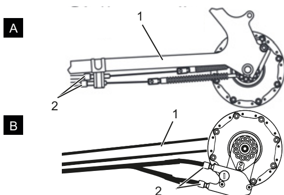
Rysunek 142: Nakrętki regulacyjne (2) w dwóch alternatywnych wersjach (A i B) dwuczętnowego mechanizmu zmiany przerzutek na rurze dolnej tylnego trójkąta (1)
