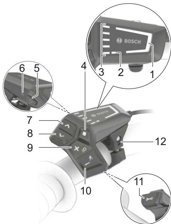
Rysunek 121: Zestawienie opcji panelu obsługi BOSCH LED Remote
