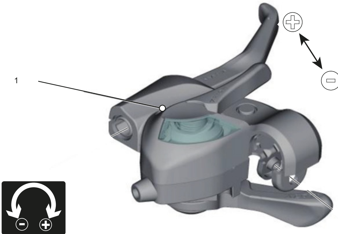
Rysunek 95: Pozycja śruby regulacyjnej (1)
