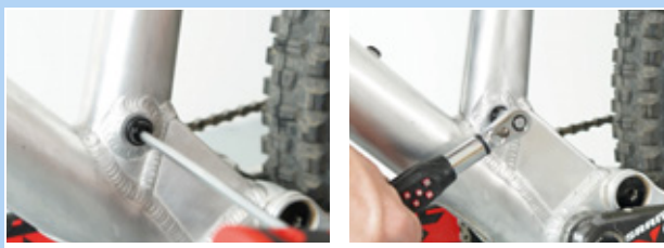
Rysunek 208: Dokręcanie sztycy podsiodłowej
