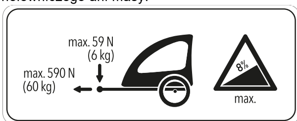
Rysunek 111: Tabliczka informacyjna przyczepki
