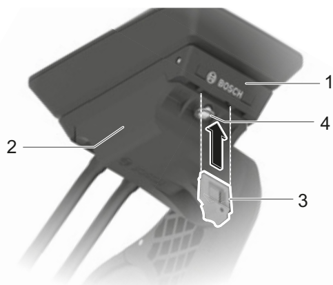
Rysunek 108: Usytuowanie śruby zespołu sterowania
