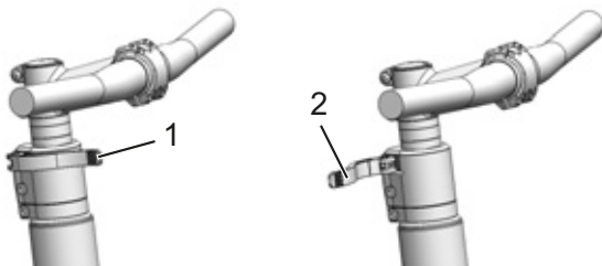
Rysunek 80: Zamknięta (1) i otwarta (2) dźwignia mocująca mostek; przykład – system regulacji All Up
